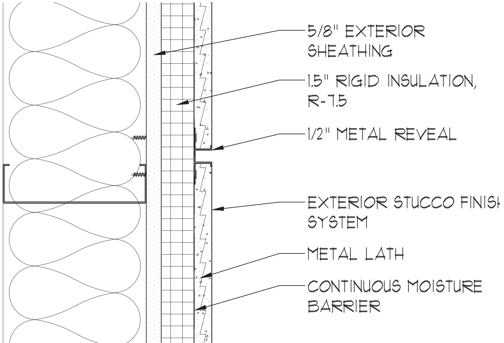
E A3.1 STUCCO CONTROL JOINT SCALE: 3" 1'-0"
